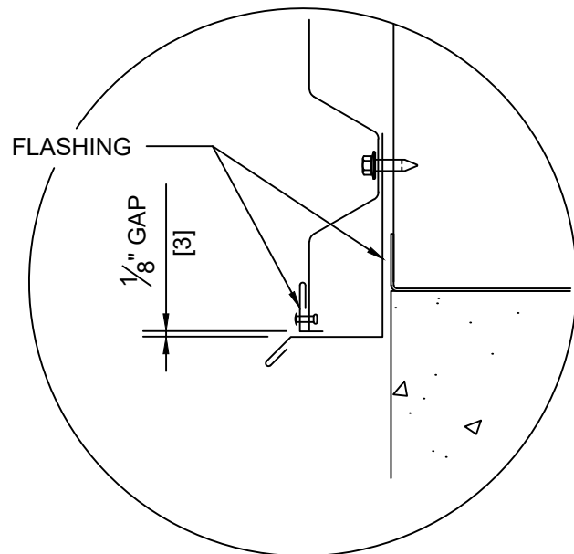
OPTIONAL DETAIL
