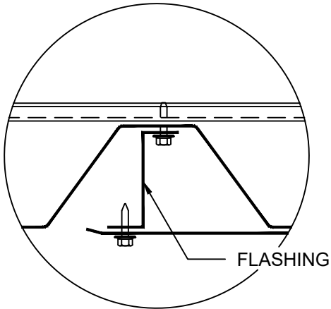
OPTIONAL LOW CELL DETAIL
