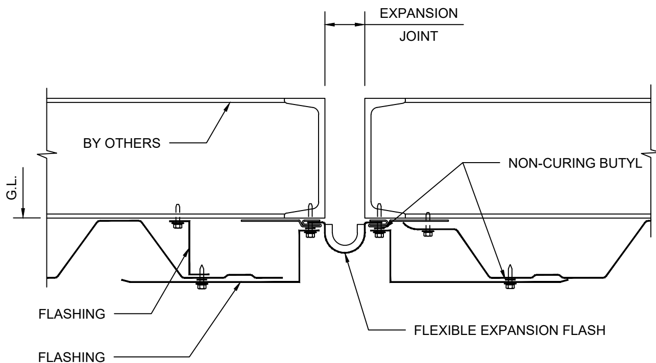
OPTIONAL LOW CELL DETAIL
