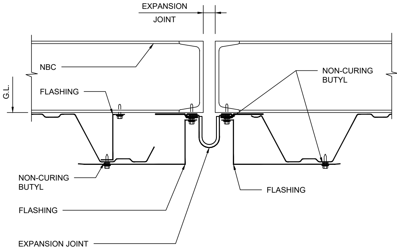
OPTIONAL LOW CELL DETAIL
