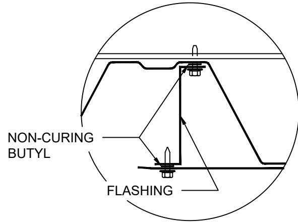
OPTIONAL LOW CELL DETAIL
