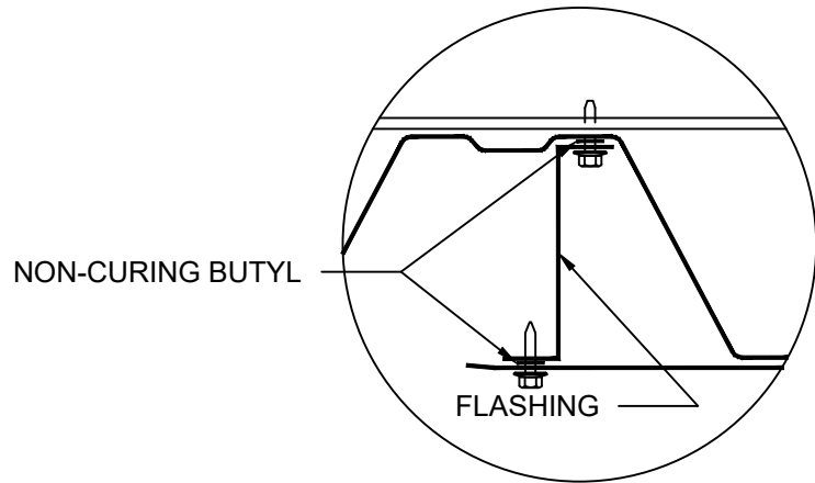
OPTIONAL LOW CELL DETAIL
