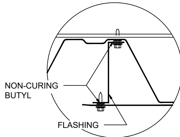
OPTIONAL LOW CELL DETAIL
