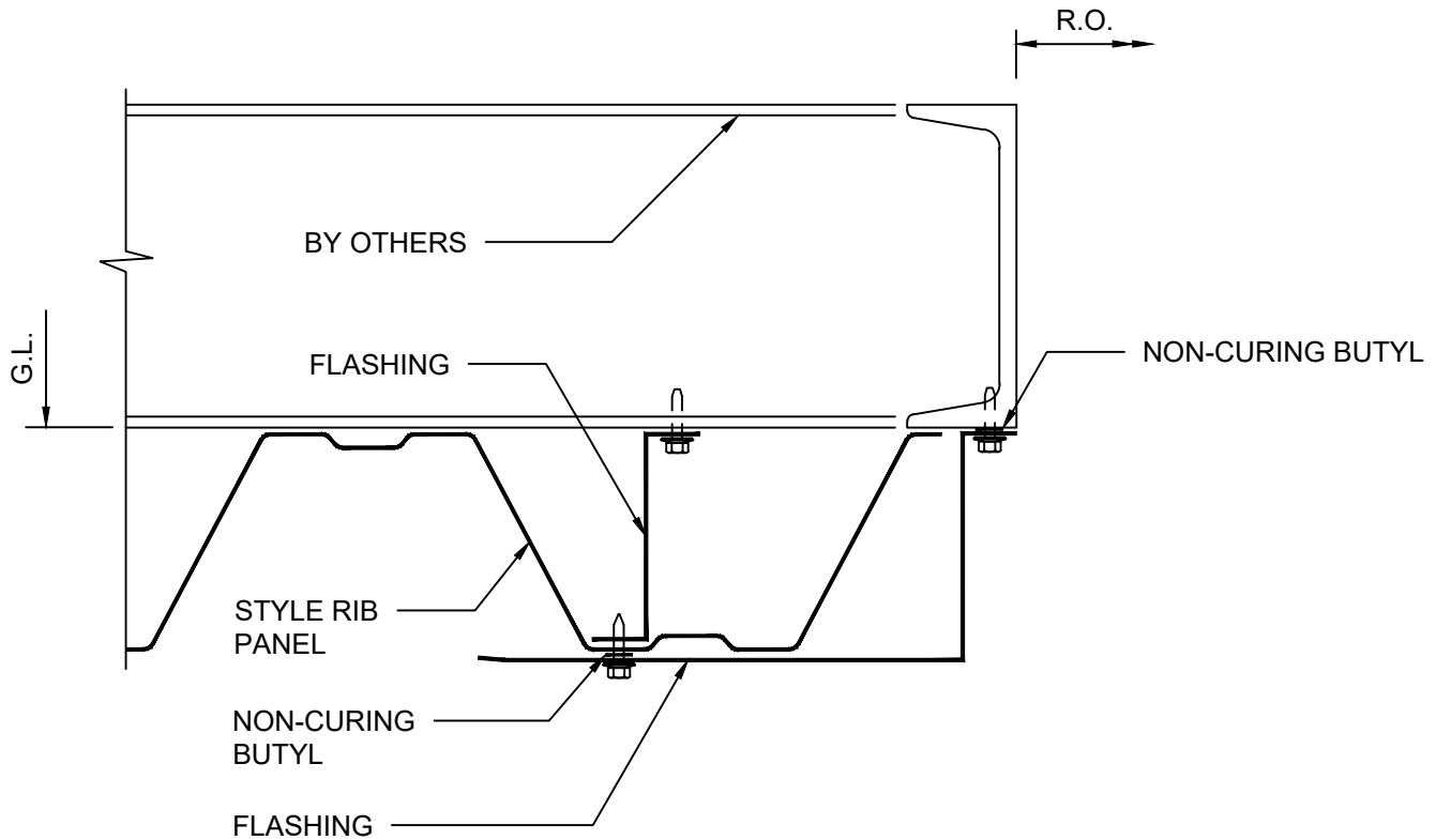
OPTIONAL LOW CELL DETAIL
