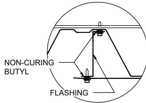
OPTIONAL LOW CELL DETAIL
