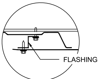
OPTIONAL LOW CELL DETAIL
