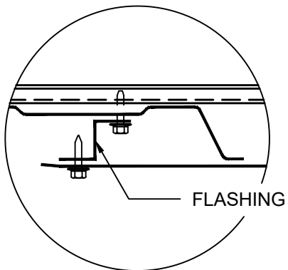
OPTIONAL LOW CELL DETAIL
