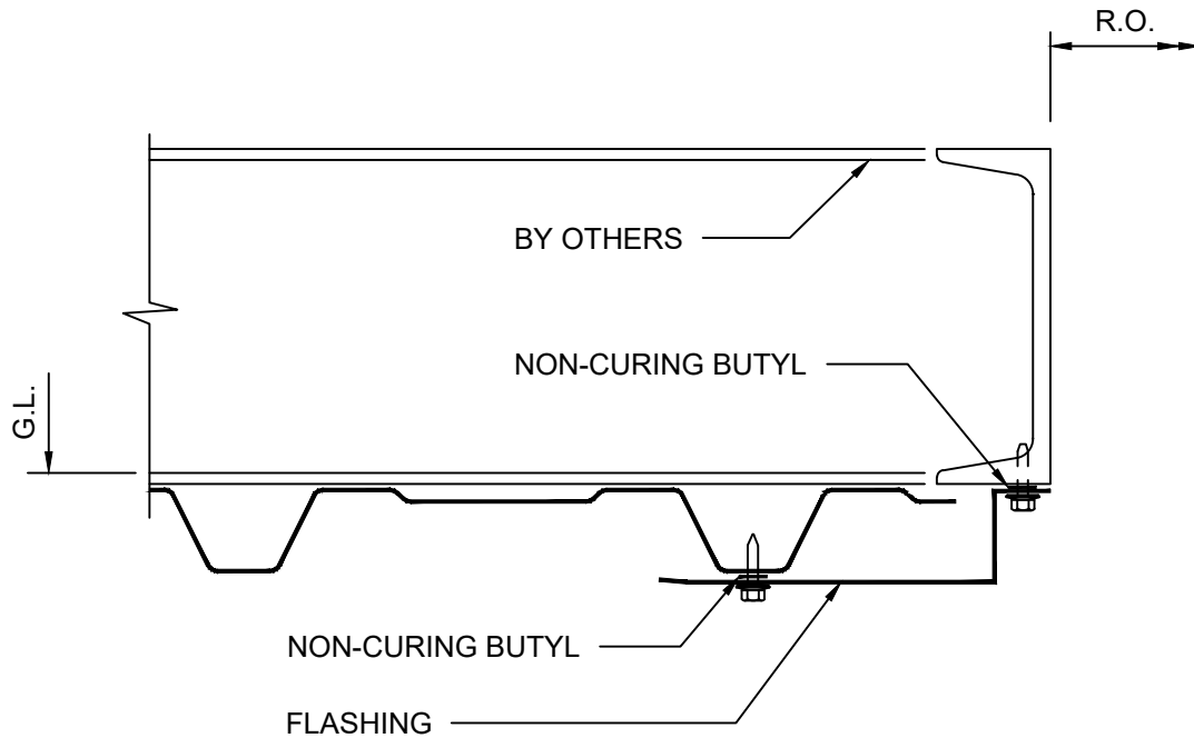
OPTIONAL LOW CELL DETAIL
