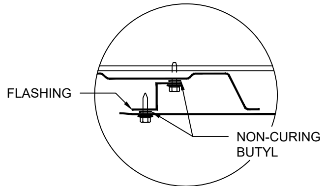
OPTIONAL LOW CELL DETAIL
